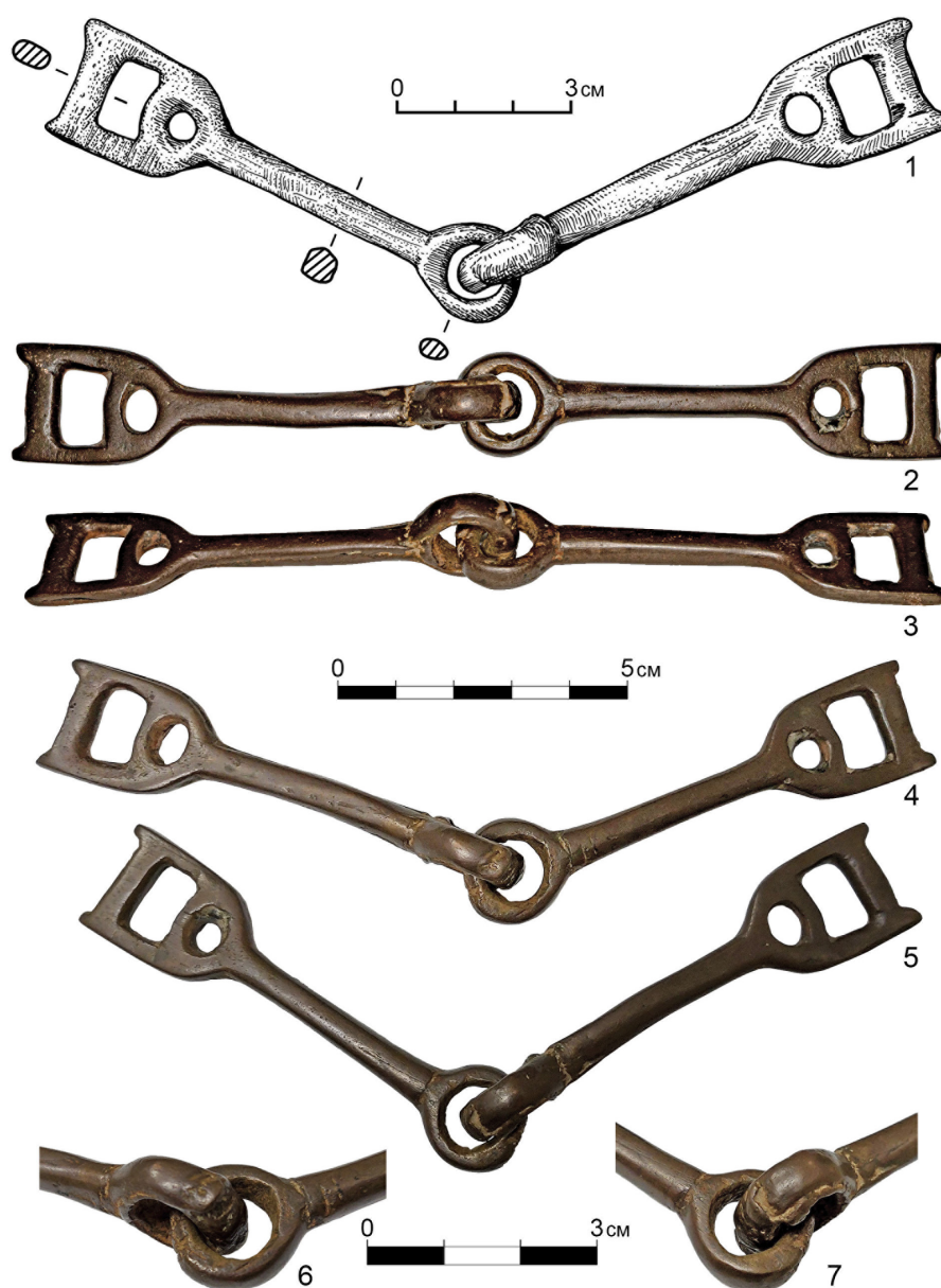
Рис. 5. Кичи-Ача, объект № 7. Бронзовые удила из клада с гладкими грызлами Fig. 5. Kichi-Acha, item No. 7. Bronze bits with smooth mouthpieces from the treasure
