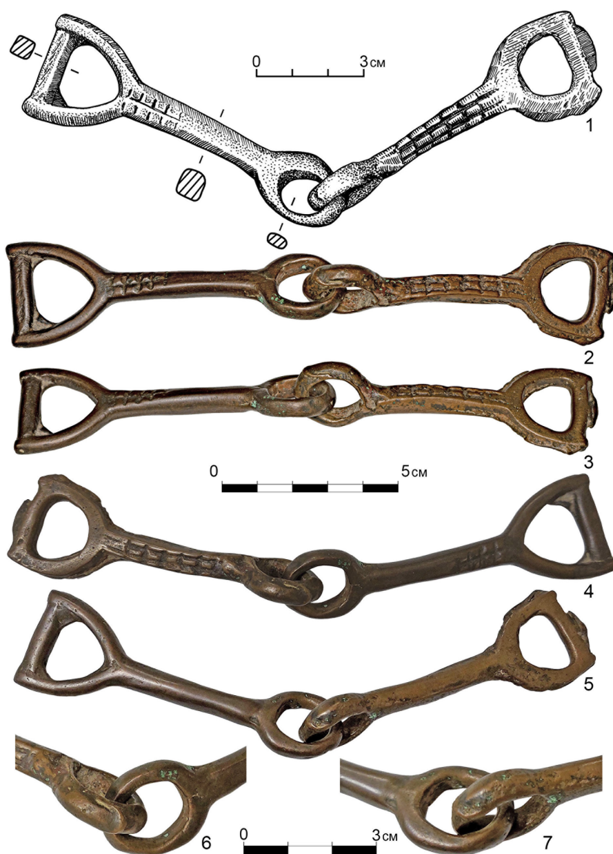
Рис. 4. Кичи-Ача, объект № 7. Бронзовые удила из клада с орнаментированными гызлами Fig. 4. Kichi-Acha, item No. 7. Bronze bits with ornamented mouthpieces from the treasure
